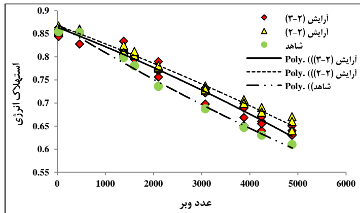
شکل ۴- تغییرات استهلاک نسبی انرژی- عدد وبر. اختلاف استهلاک انرژی برای آرایش متفاوت موانع نسبت به مدل شاهد
