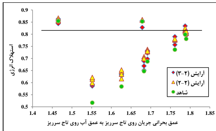
شکل ۳- تغییرات استهلاک نسبی انرژی - y/H . اختلاف استهلاک انرژی برای آرایش متفاوت موانع نسبت به مدل شاهد
