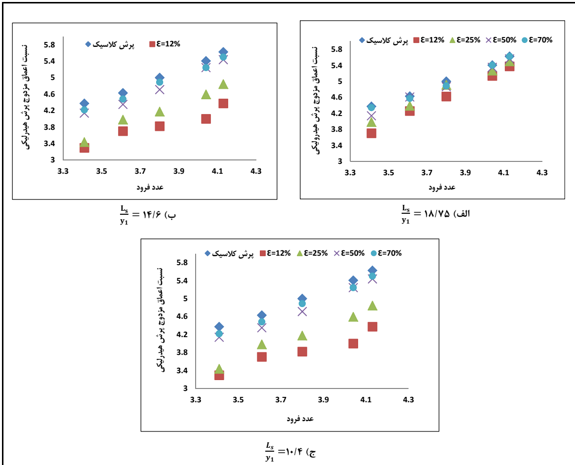
شکل ۹- تغییرات نسبت اعماق مزدوج پرش هیدرولیکی در فاصله‌های نسبی مختلف
