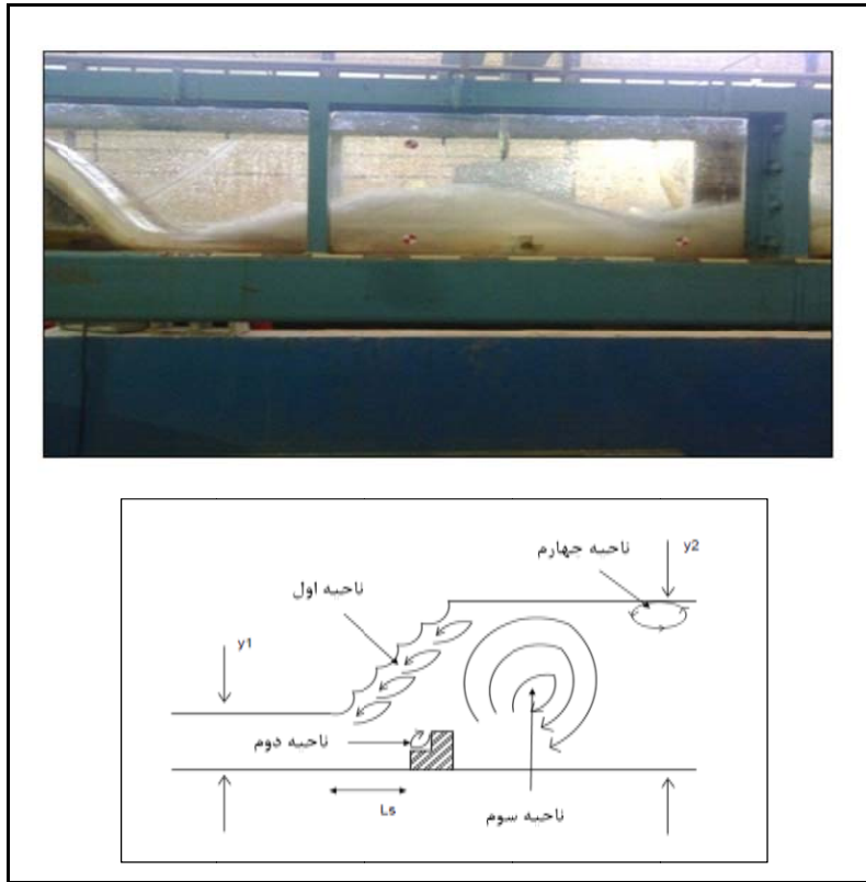
شکل ۵- انواع گرداب تشکیل شده در حوضچه آرامش ( Q = 35/53 \frac{L^3}{s} و \frac{L_j}{y_1} = 14/6 )
