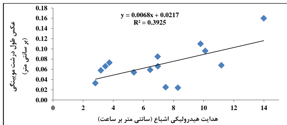
شکل ۵- روند تغییرات مقدار طول درشت موئینی خاک نسبت به هدایت هیدرولیکی اشباع خاک
