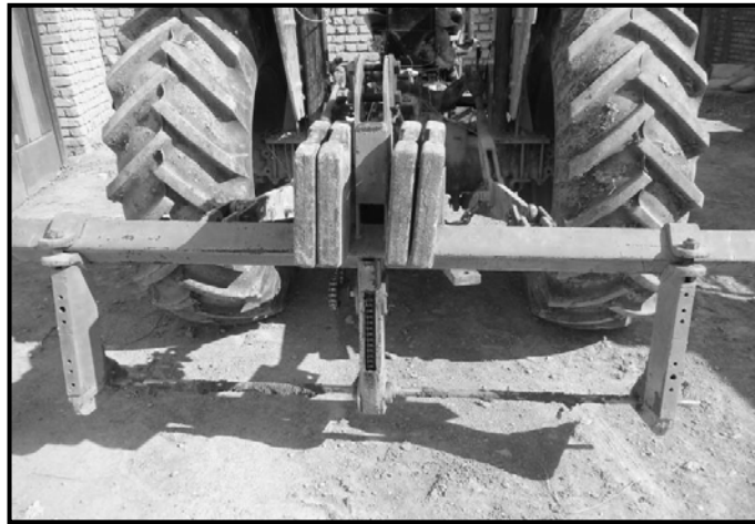
شکل ۵- پیازکن میله‌ای در حالت عقب‌سوار با وزنه‌های سنگین‌کننده
