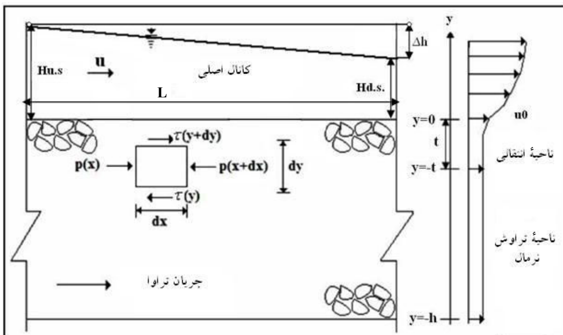
شکل ۱- نمایشی از جریان از درون و روی سد سنگریزه‌ای تأخیری در حالت استغراق
