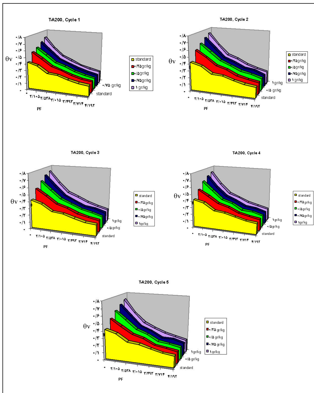
شکل ۲- منحنی رطوبتی خاک- پلیمر T-A200 در تیمارهای ۰، ۲۵، ۵۰، ۷۵ و ۱ گرم پلیمر بر کیلوگرم خاک در هر سیکل متوالی در خاک لوم
