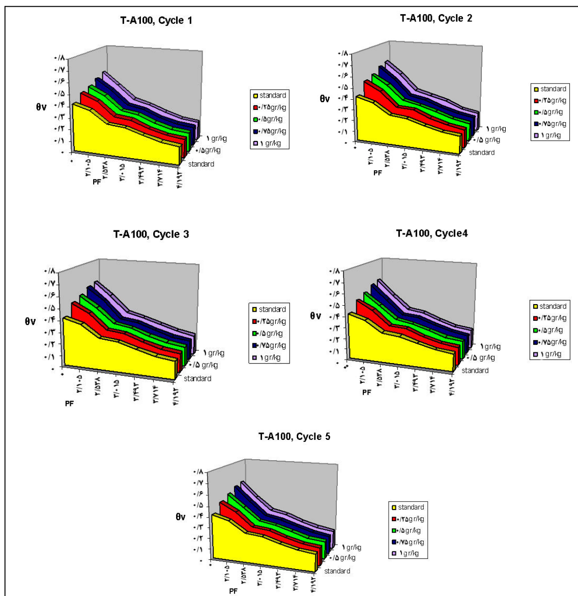
شکل ۳- منحنی رطوبتی خاک- پلیمر T-A100 در تیمارهای
