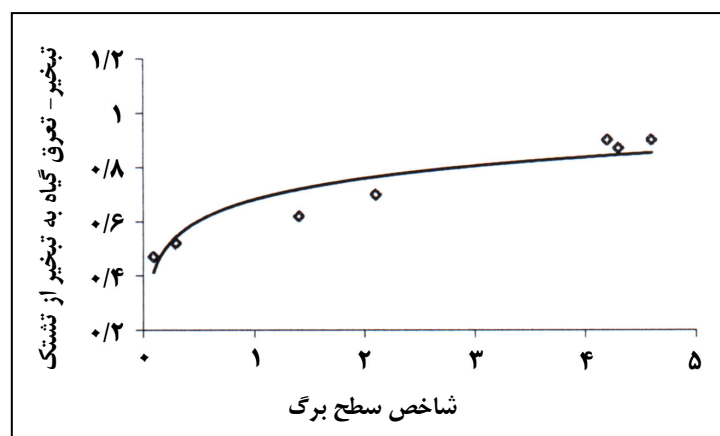
شکل شماره ۱۱- تغییرات "تبخیر تعرق گیاه به تبخیر از تشتک" نسبت به شاخص سطح برگ
