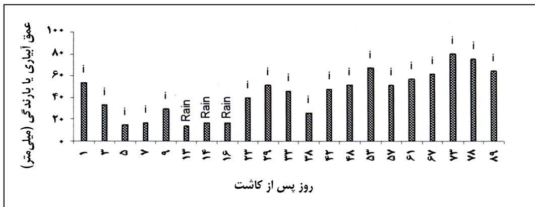
شکل شماره ۲- زمان و مقدار آبیاری و بارندگی در تیمار آبیاری کامل
