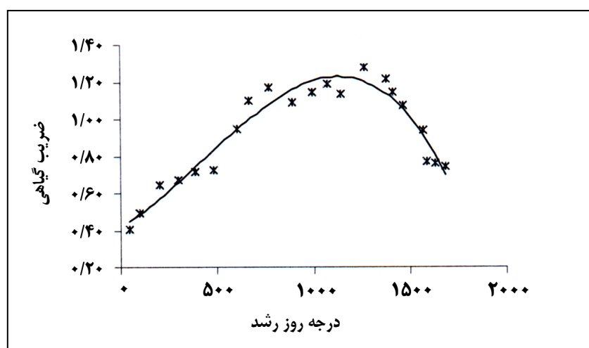
شکل شماره ۸- تغییرات ضریب گیاهی نسبت به درجه روز رشد (GDD)
