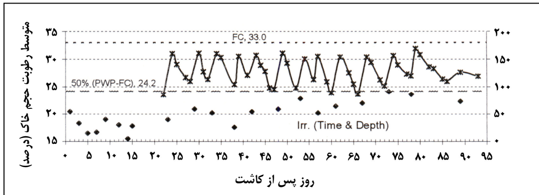
شکل شماره ۱- تغییرات رطوبت نیمرخ خاک در عمق ۶۰ سانتی‌متری در طول فصل رشد در تیمار بیش آبیاری
