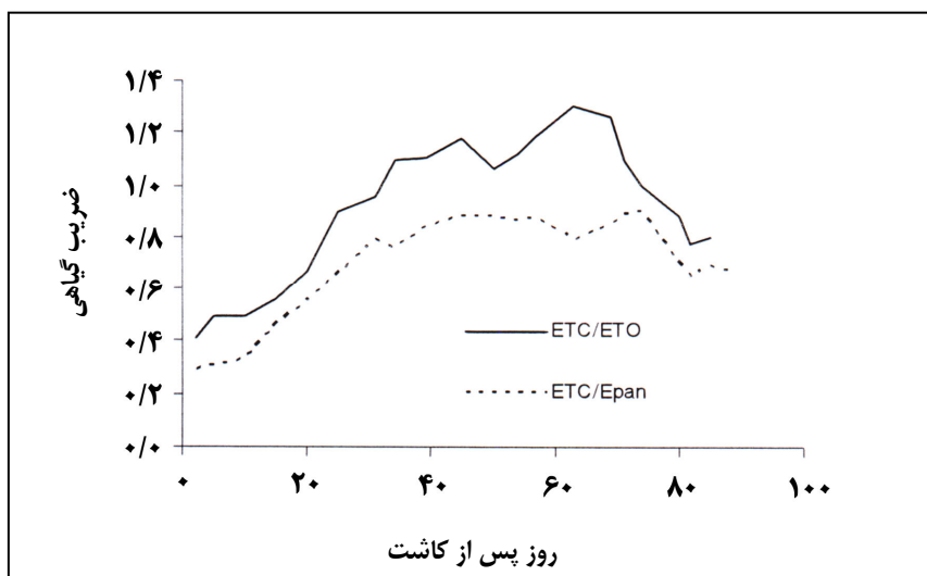
شکل شماره ۴- تغییرات ضریب گیاهی ( K_c ) و نسبت ET_c/E_{pan} ذرت علوفه‌ای طی دوره رشد
