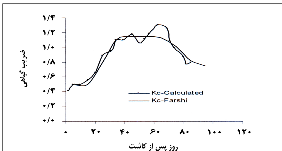
شکل شماره ۶- مقایسه ضریب گیاهی ذرت دانه‌ای و ذرت علوفه‌ای ( K_{c-calc} )
