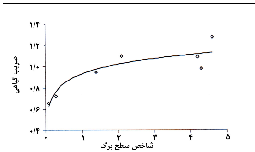
شکل شماره ۹- تغییرات ضریب گیاهی نسبت به شاخص سطح برگ
