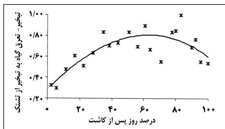
شکل شماره ۱۰- تغییرات "تبخیر - تعرق گیاه به تبخیر از تشتک" نسبت به درصد دوره رشد ( DASP )
