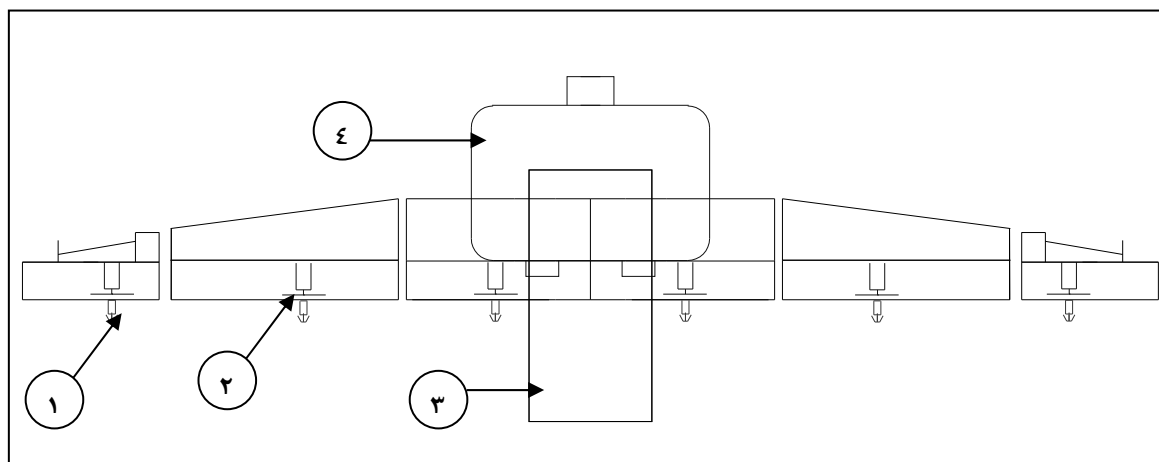
شکل شماره ۱- تصویر شماتیک از سمپاش بوم دار تراکتوری مجهز به صفحات چرخان (دید از جلو) ۱- فنجان دوار ۲- دمنده ۳- شاسی ۴- مخزن
