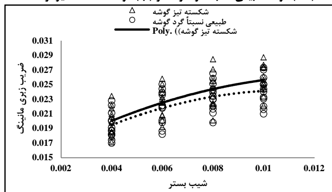
شکل ۵- تغییرات ضریب زبری مایننگ در مقابل شیب بستر برای ذرات شکسته تیز گوشه و ذرات طبیعی نسبتاً گرد گوشه
