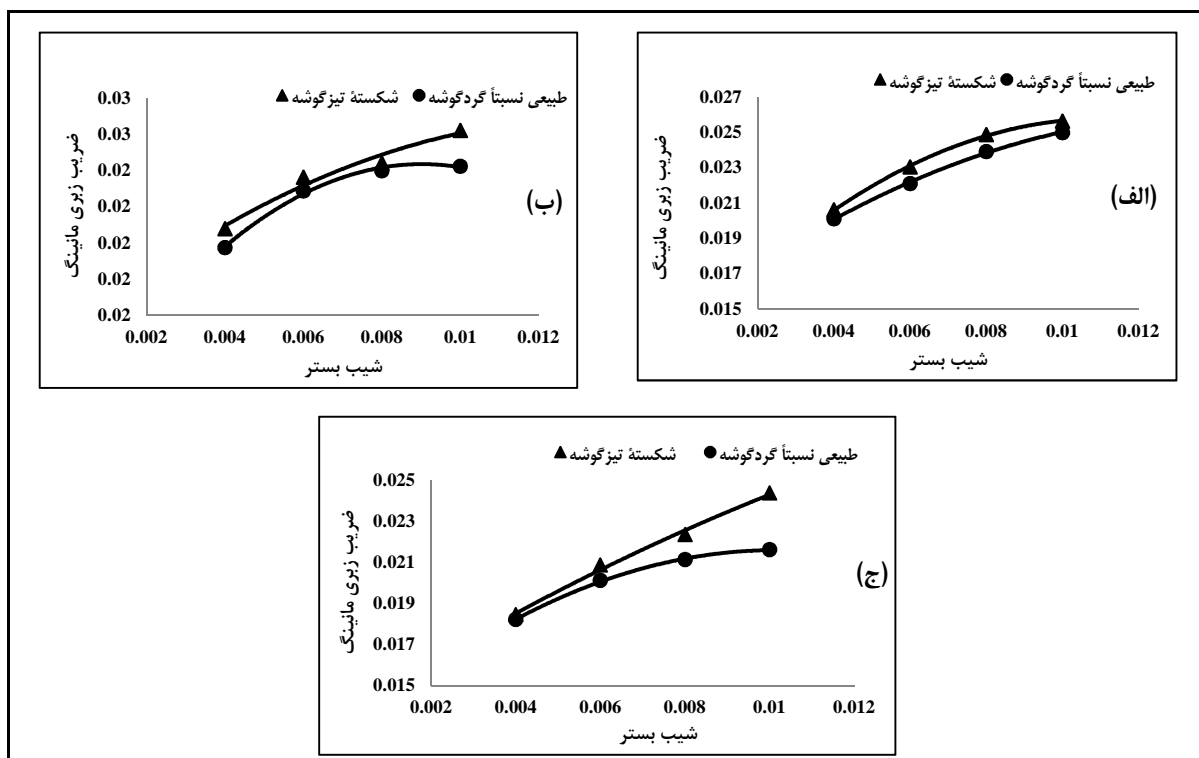
شکل ۳- تغییرات ضریب زبری مایننگ در مقابل شیب بستر به ازای دبی ثابت ۲۴ لیتر در ثانیه برای:
