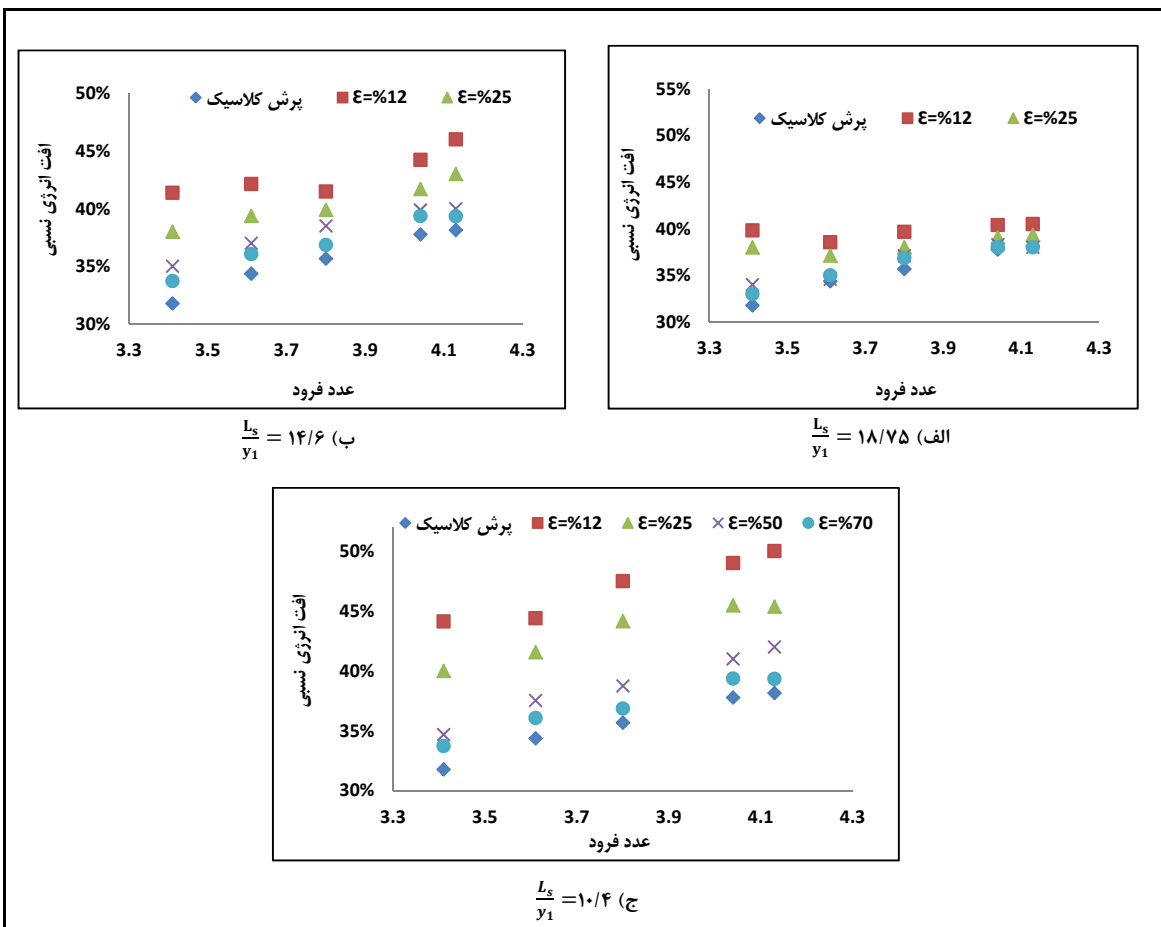
شکل ۱۰- تغییرات افت انرژی نسبی پرش هیدرولیکی به‌ازای عدد فرود در فاصله‌های نسبی مختلف
