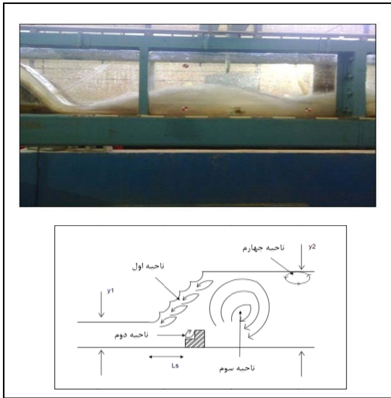
شکل ۵- انواع گرداب تشکیل شده در حوضچه آرامش ( Q = 35/53 \frac{L^3}{s} و \frac{L_s}{y_1} = 14/6 )
