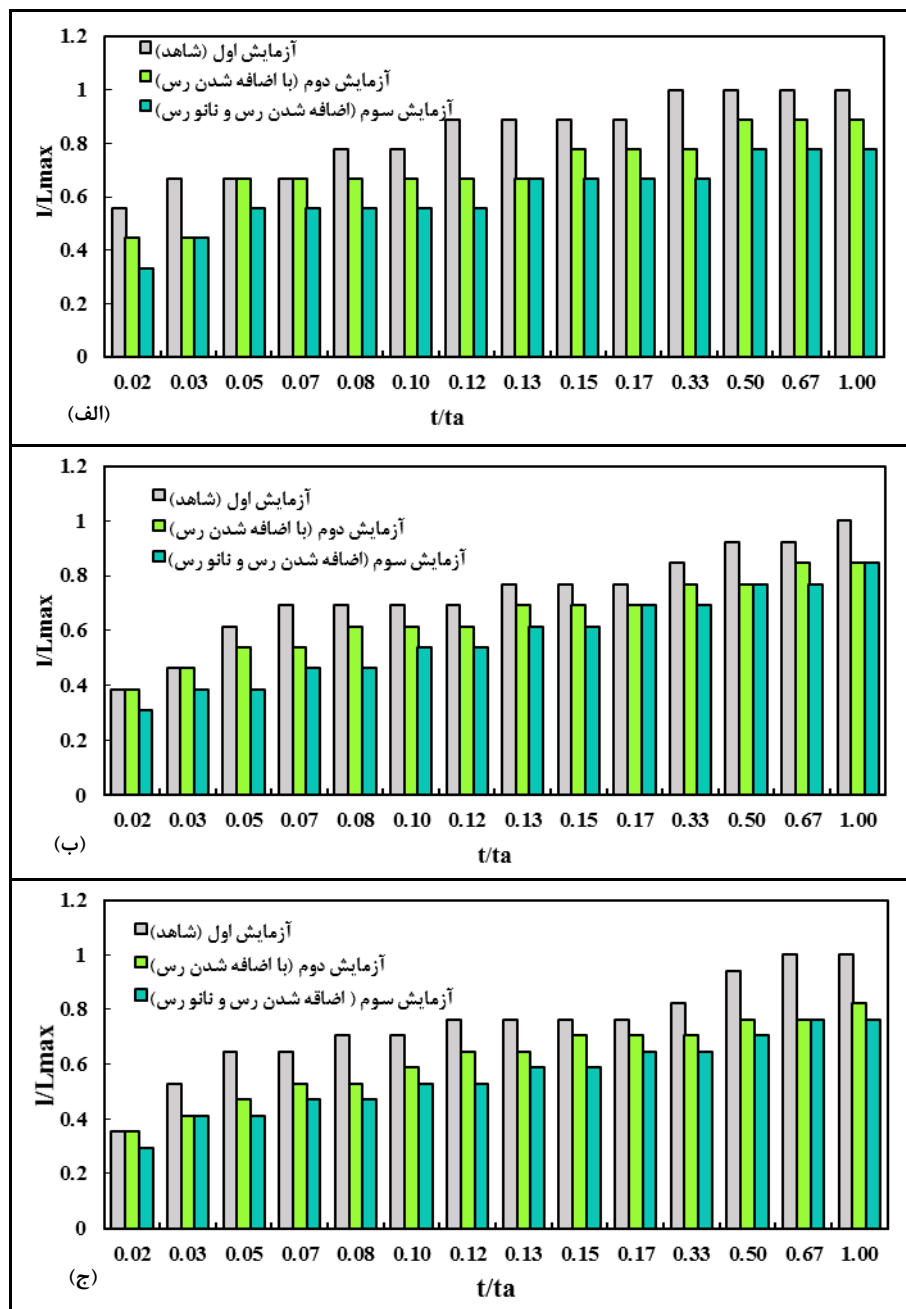
شکل ۷- تغییرات زمانی طول نسبی آبشستگی با اضافه شدن رس و ترکیب آن با نانو رس مونت موریلونیتی
