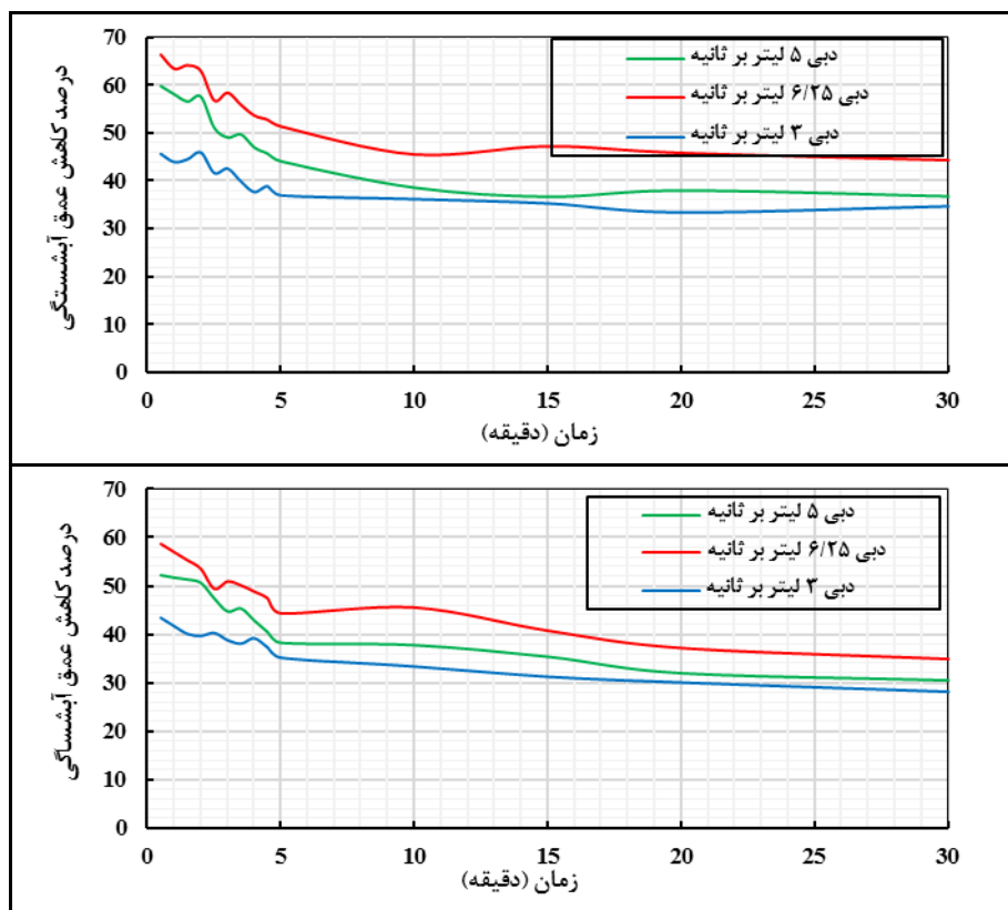
شکل ۸- نمودار تغییرات زمانی درصد کاهش عمق آبستگي ناشی از اضافه شدن رس (الف) رس به ذرات رسوبی و ب) ترکیب رس و نانو رس مونت موریلونیتی به ذرات رسوبی
