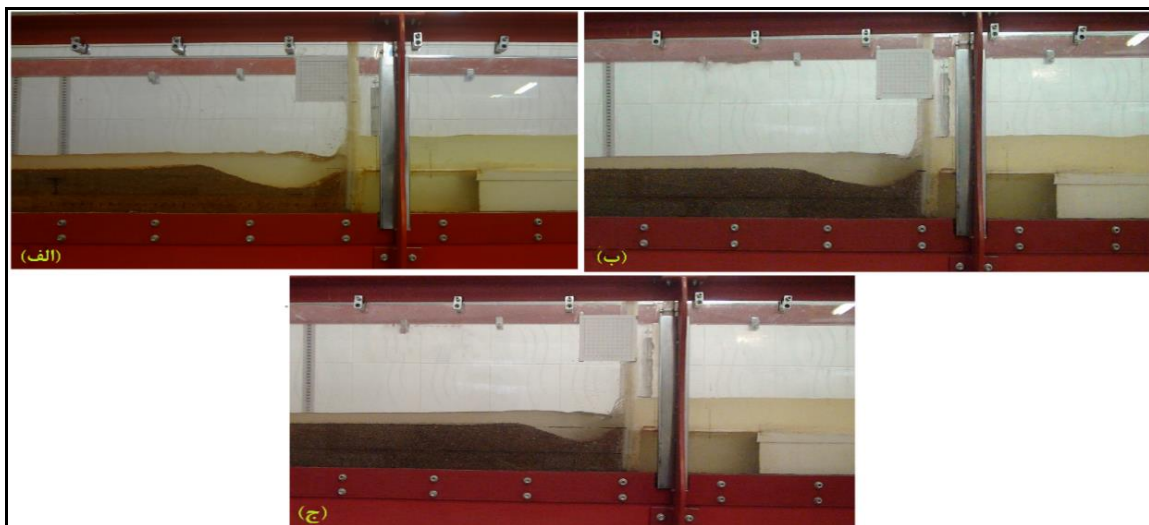
شکل ۱۰- نمایی از پروفیل طولی آبشستگی
