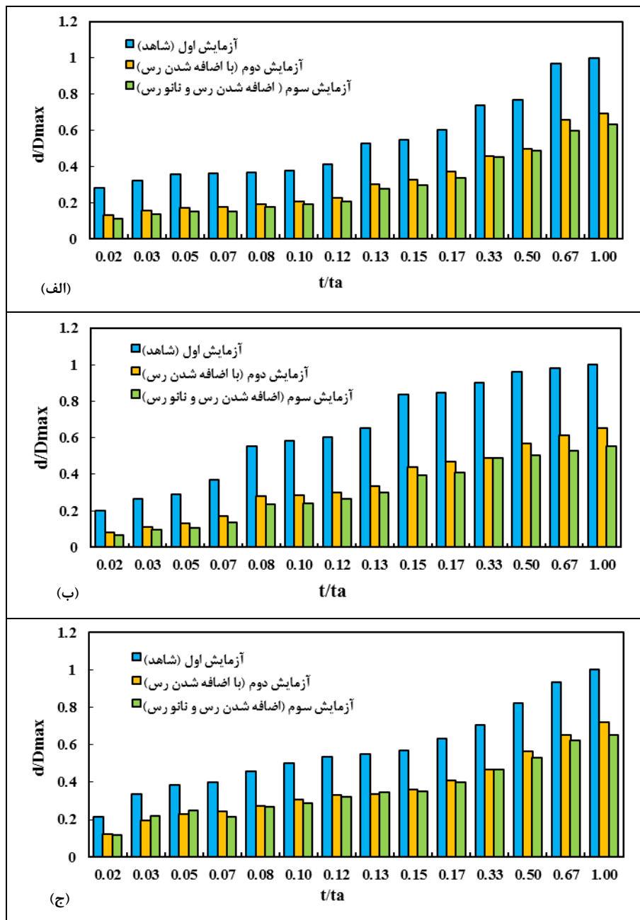
شکل ۶- تغییرات زمانی عمق نسبی آبستگي با اضافه شدن رس و ترکیب آن با نانو رس مونت موریلونیتی
