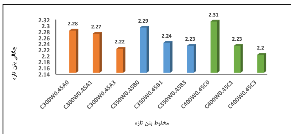
شکل ۵- مقادیر چگالی بتن تازه در مخلوط‌های مختلف
