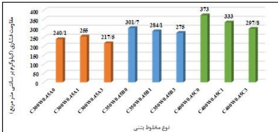
شکل ۶- مقدار مقاومت فشاری آزمون‌های مخلوط‌های مورد آزمایش
