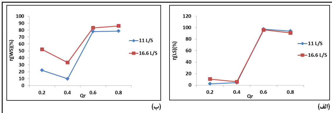
شکل ۷- مقدار کاهش الف) طول جدانشدگی و ب) عرض جدانشدگی جریان در حالت گردگوشه نسبت به تیزگوشه
