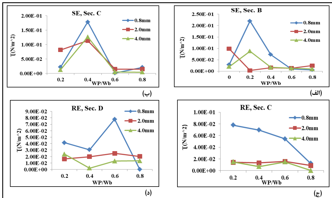
شکل ۱۰- مقایسه تنش برشی در زبری‌های مختلف الف) مقطع B و حالت تیزگوشه، ب) مقطع C و حالت تیزگوشه، ج) مقطع C و حالت گردگوشه و د) مقطع D و حالت گردگوشه
