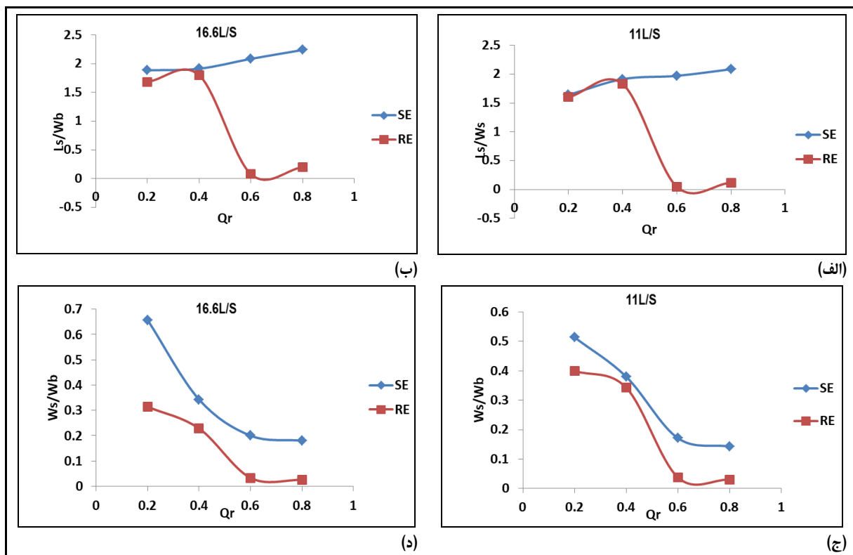
شکل ۶- مقایسه بین ابعاد جداولدگی در حالت تیز گوشه و گرد گوشه
