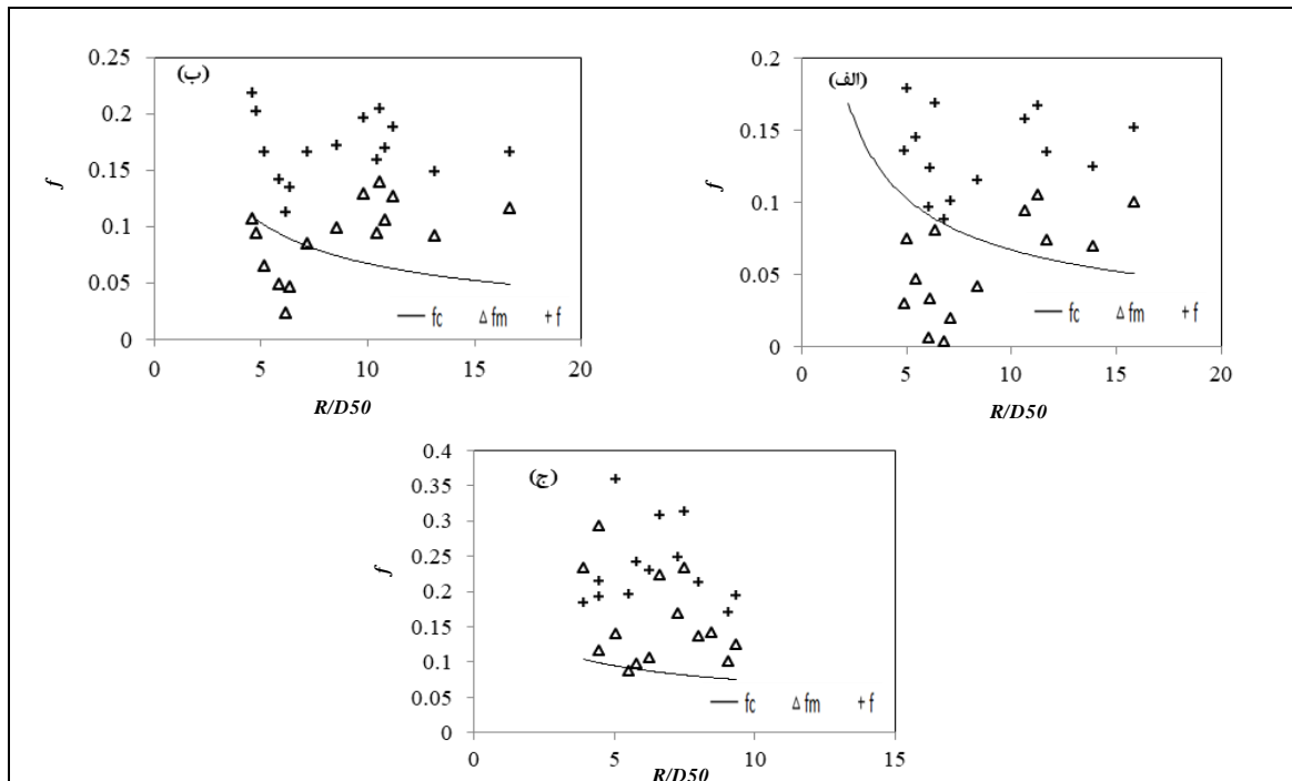
شکل ۶- تغییرات ضریب اصطکاک f و f_m نسبت به R/D بر اساس تئوری خطی برای حالت‌های الف) شیب ۲ درصد، ب) شیب ۳ درصد و ج) شیب ۵ درصد
