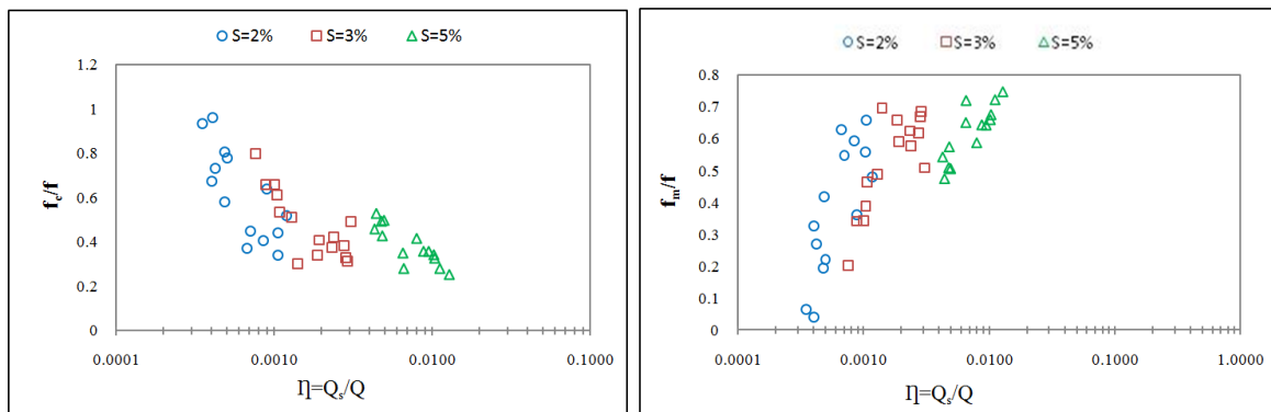
شکل ۷- تأثیر شیب بر ضریب f_m/f و f/f_m نسبت به میزان جابه‌جایی بار بستر ۷
