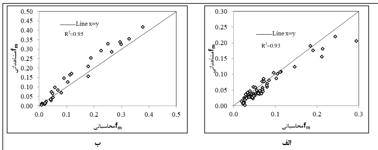
شکل ۱۰- مقایسه رابطه پیشنهادی این تحقیق (رابطه ۱۶) با نتایج آزمایشگاهی اسمارت و جگی (Smart & Jaeggi, 1983) و کائو (Cao, 1985)
