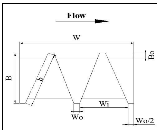
شکل ۴- نحوه قرارگیری سرریز به حالت ۱
