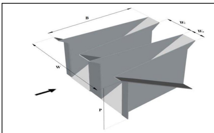
شکل ۲- نمایی از سرریز کلید پیانویی دوزنقه‌ای تیپ A (Mehboudi et al. , 2016)
