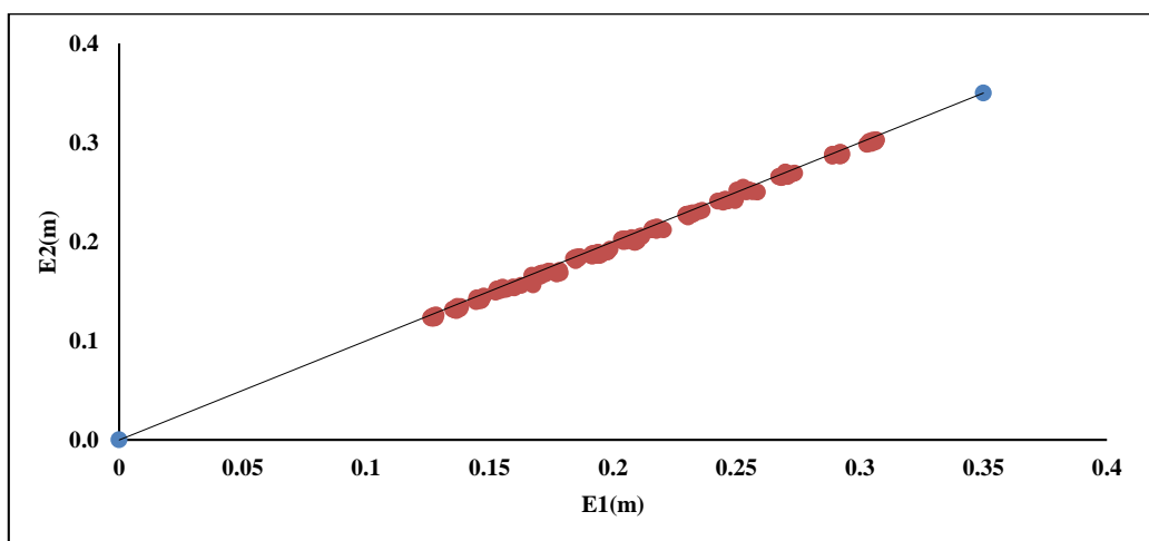
شکل ۱۷- انرژی اولیه و ثانویه سرریز Fig. 17- Primary and secondary energies of the weir
