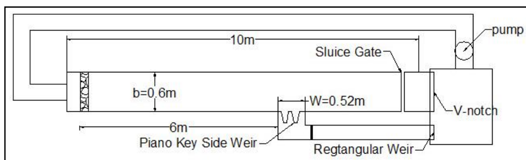
شکل ۵- نمایی از پلان شرایط آزمایشگاه
