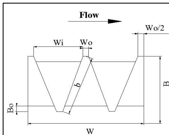
شکل ۳- نحوه قرارگیری سرریز به حالت ۲
