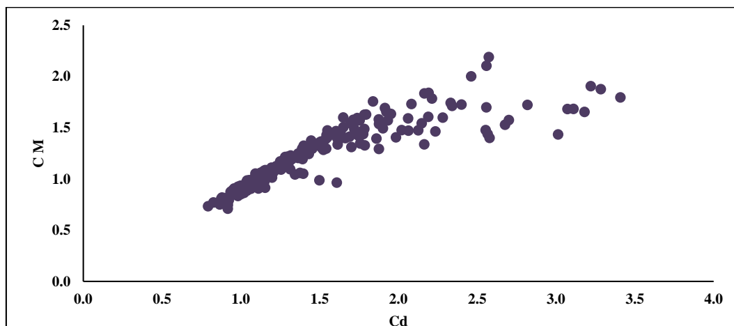
شکل ۱۸- ضرایب دبی C_d و C_M Fig. 18- Discharge coefficients of C_d and C_M
