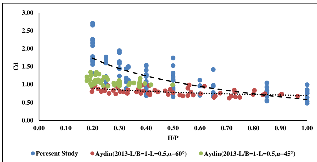
شکل ۱۶- مقایسه ضریب دبی عبوری سرریز کلید پیانویی دوزنقه‌ای و مثلثی و سرریز کنگره‌ای مثلثی Fig. 16- Comparison between the discharge coefficients of the labyrinth triangular side weir and side trapezoidal piano key weir
