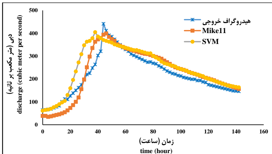
شکل ۵- هیدروگراف خروجی مشاهداتی و محاسباتی توسط مدل‌های Mike11 و SVM برای مرحله صحت‌سنجی (تاریخ ۱۳۷۹/۰۱/۰۵) Fig. 5- Observational and computational output hydrographs by Mike11 and SVM models for validation (date 2000/03/24)
