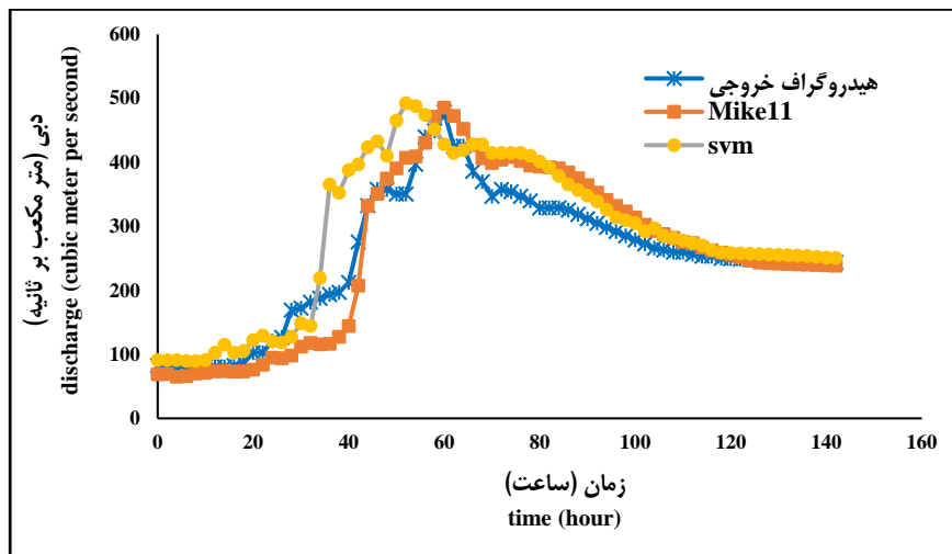
شکل ۴- هیدروگراف خروجی مشاهداتی و محاسباتی توسط مدل‌های Mike11 و SVM برای مرحله صحت‌سنجی (تاریخ ۱۳۶۳/۰۹/۰۳) Fig. 4- Observational and computational output hydrographs by Mike11 and svm models for validation (date 1984/11/23)
