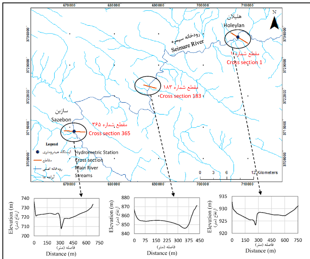
شکل ۱- محدوده مطالعاتی واقع بر رودخانه سیمره (بازه هلیلان تا سازبن) و موقعیت برخی مقاطع رودخانه ای مورد استفاده
