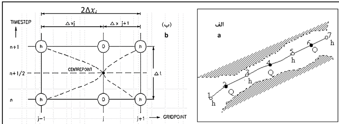
شکل ۲- الف) روش حل معادلات در نرم‌افزار MIKE11 و ب) شبکه شش نقطه‌ای ابوت مربوط به معادلات پیوستگی و مومنتوم Fig. 2- a) Method of solving equations in MIKE11 software, b) Abbott's six-point network for the continuity and momentum equations
