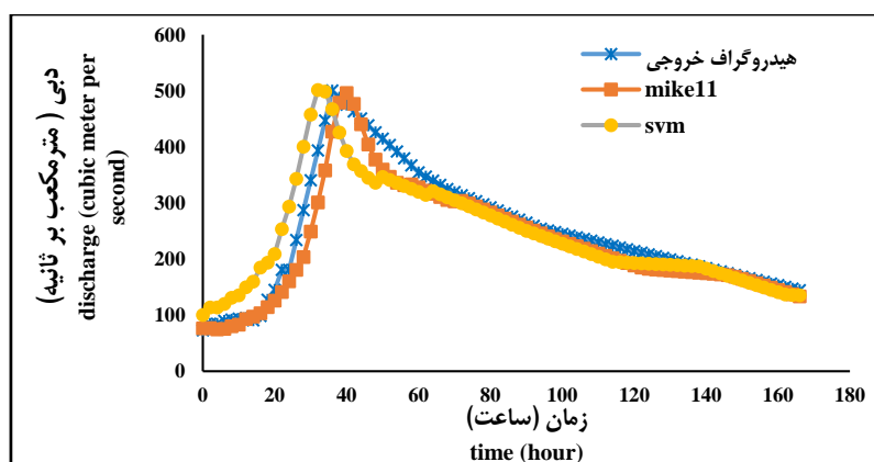
شکل ۳- هیدروگراف خروجی مشاهداتی و محاسباتی توسط مدل‌های Mike11 و SVM برای مرحله واسنجی (تاریخ ۱۳۷۱/۱۰/۱۷) Fig. 3- Observational and Computational Output Hydrograph by Mike11 and SVM Models for Calibration (date 1993/01/06)
