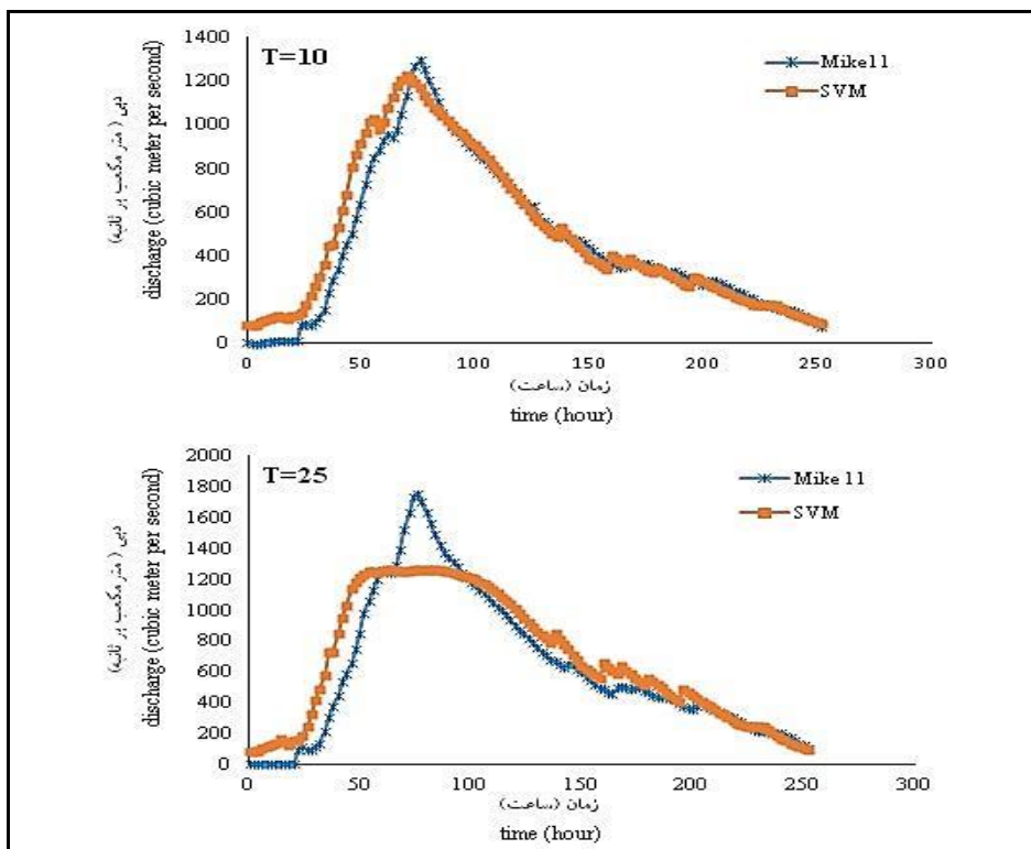
شکل ۷- هیدروگراف سیل محاسباتی با مدل Mike11 و SVM با دوره بازگشت های ۱۰ و ۲۵ سال
