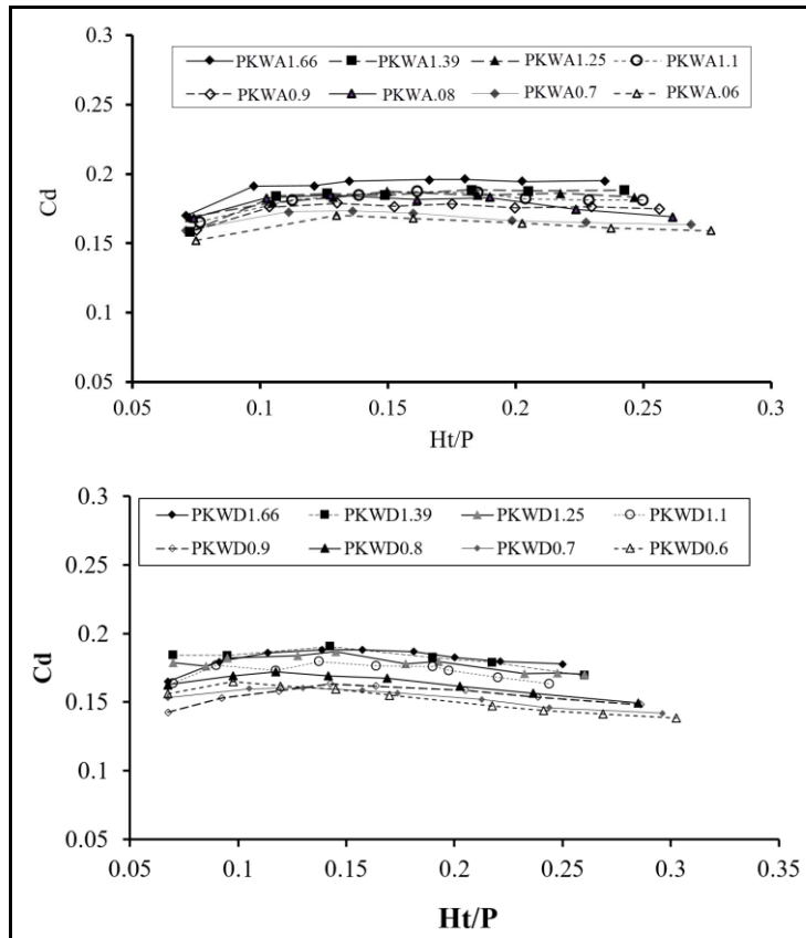
شکل ۷- نمودار تغییرات Cd در مقابل Ht/P به ازای نمای بار هیدرولیکی ۱/۳
