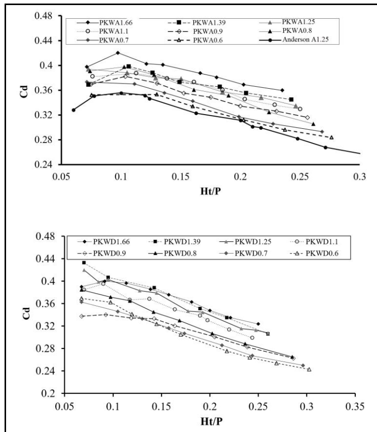
شکل ۵- تغییرات ضریب دبی سرریز نوع A (بالا) و نوع D (پایین) در مقابل بار آبی به‌ازای W_i/W_o های مختلف Fig. 5- Variations of discharge coefficient of PKW-A (top) and PKW-D (bottom) vs. flow heads for different ratios of w_i/w_o
