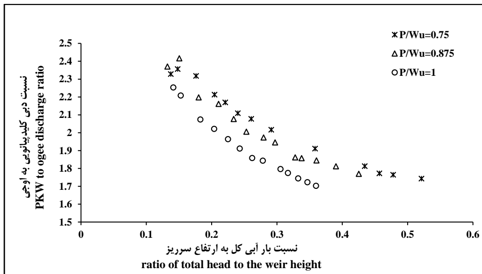
شکل ۱۰- مقایسه دبی عبوری از سرریز کلیدپیانویی و سرریز اوجی در نسبت‌های مختلف P/W_u
