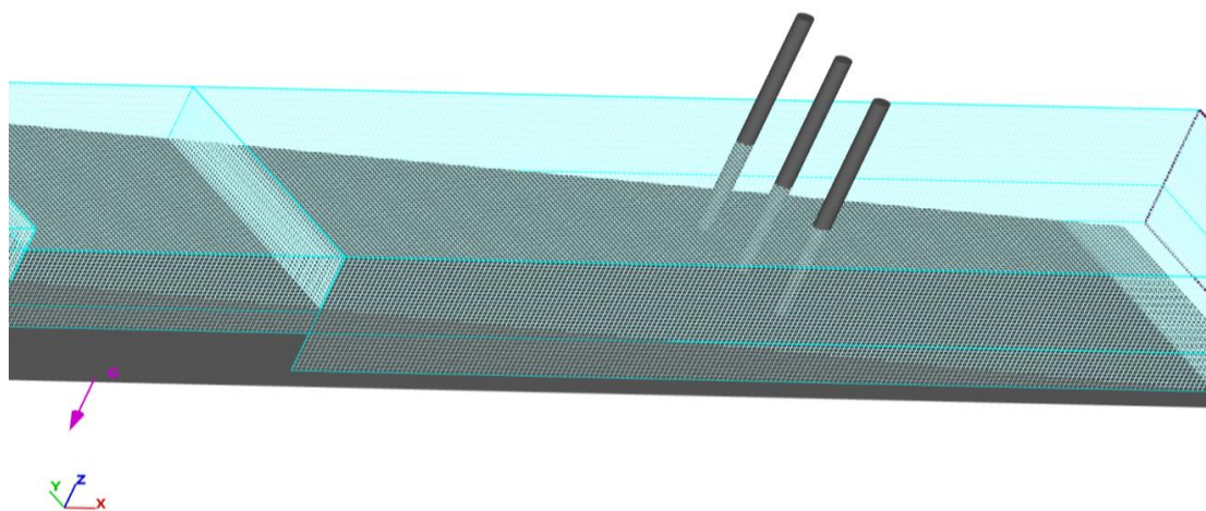
شکل ۶- نمایی از مش بندی کانال مدل‌سازی شده در نرم افزار FLOW-3D
